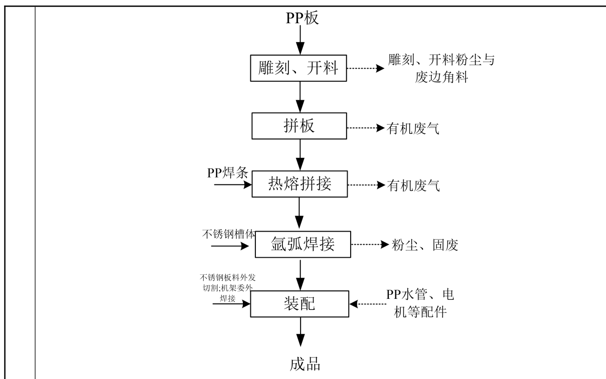
图 2-2 生产工艺流程及产污节点（PP 板）
