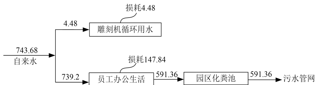
图 2-1 项目水平衡图 (单位: m 3 /a)
